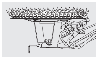
Patrón correcto de la llama del quemador y el piloto
