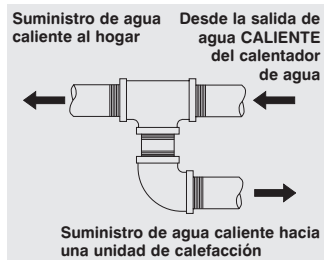
Conector en forma de T para tuberías horizontales de suministro de agua caliente
