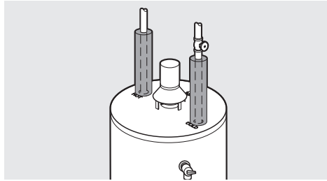
Instalación típica de tubería vertical
