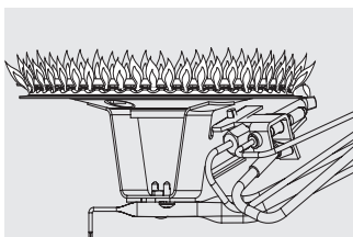
Patrón correcto del quemador principal y el quemador del piloto
